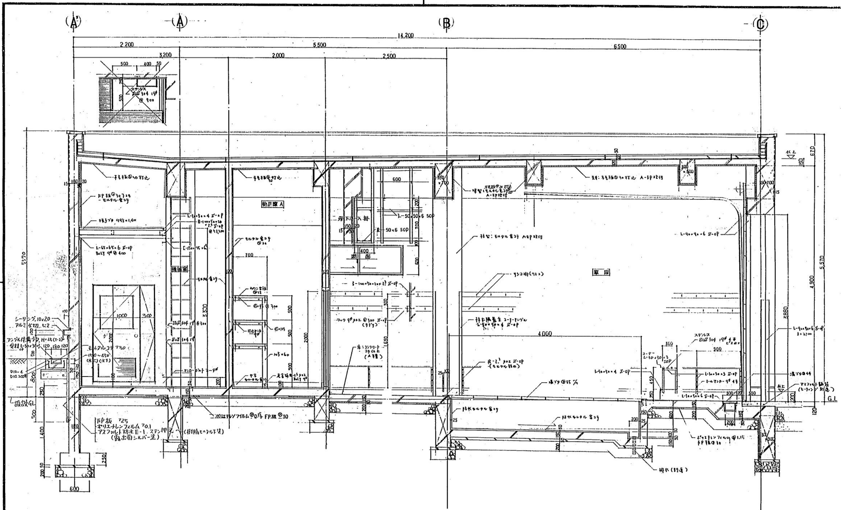
矩計図 1:30
