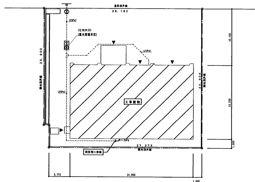
屋外配置図 S=1:200
