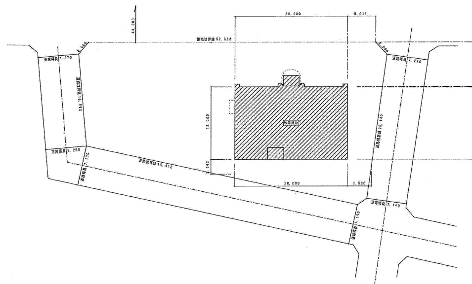
配置図 S=1/200
