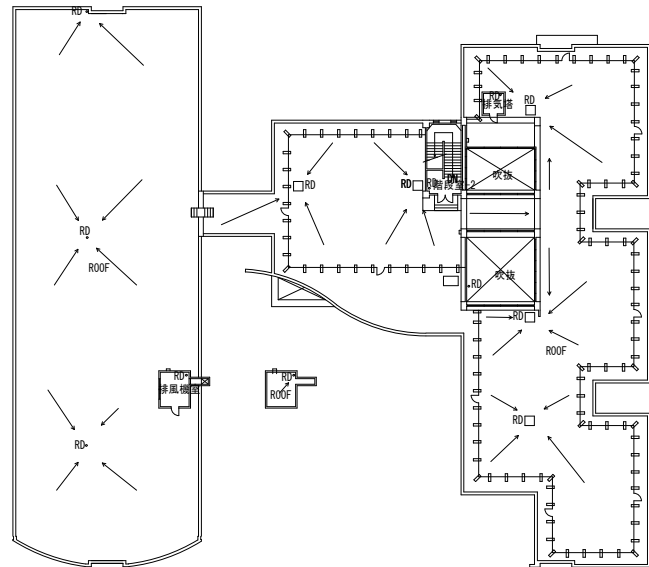
塔屋平面図 S=1:400
