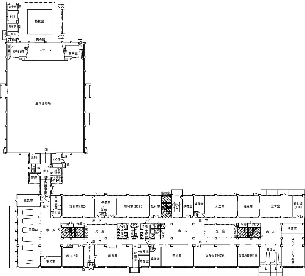
1階平面図 S=1：400
