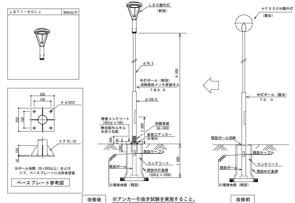
屋外灯改修図 (基礎再利用)
