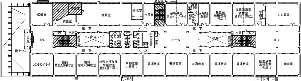
2階平面図 S=1：400
