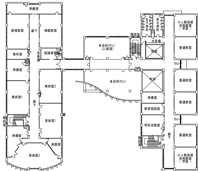
3階平面図 S=1:400
