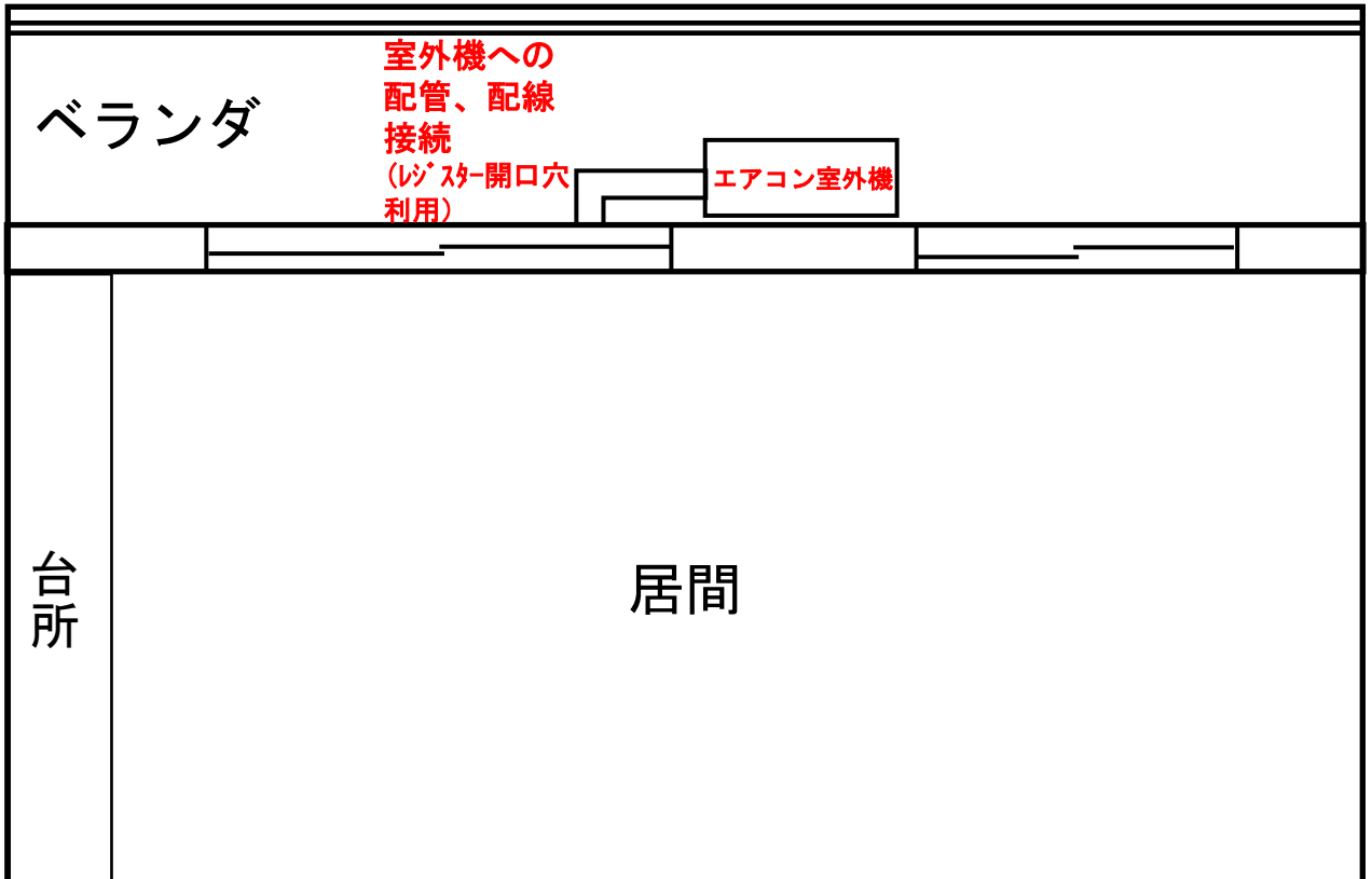
平面図（居間、ベランダ）
